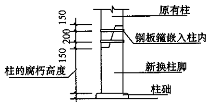
图 10.1.5 拍巴掌榫接
