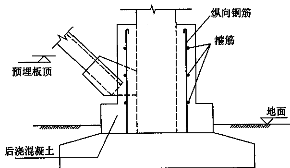
图 8.3.8 柱根部加固
