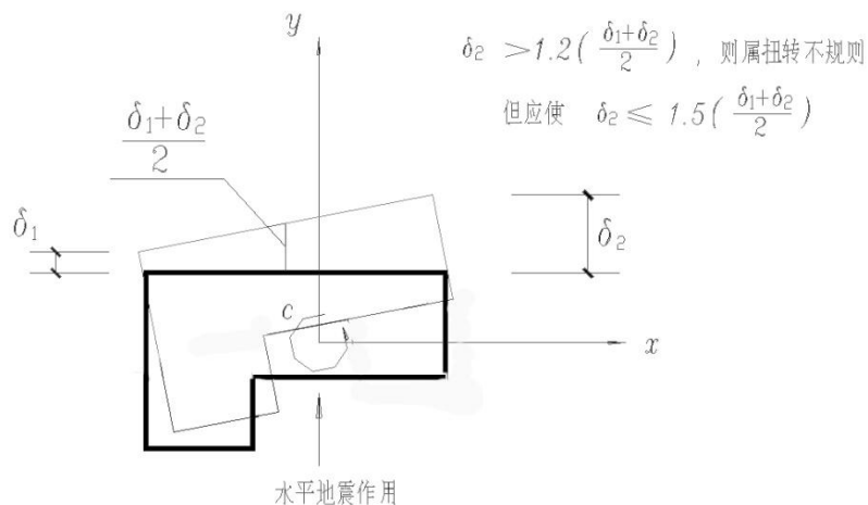
图 1 建筑结构平面的扭转不规则示例
