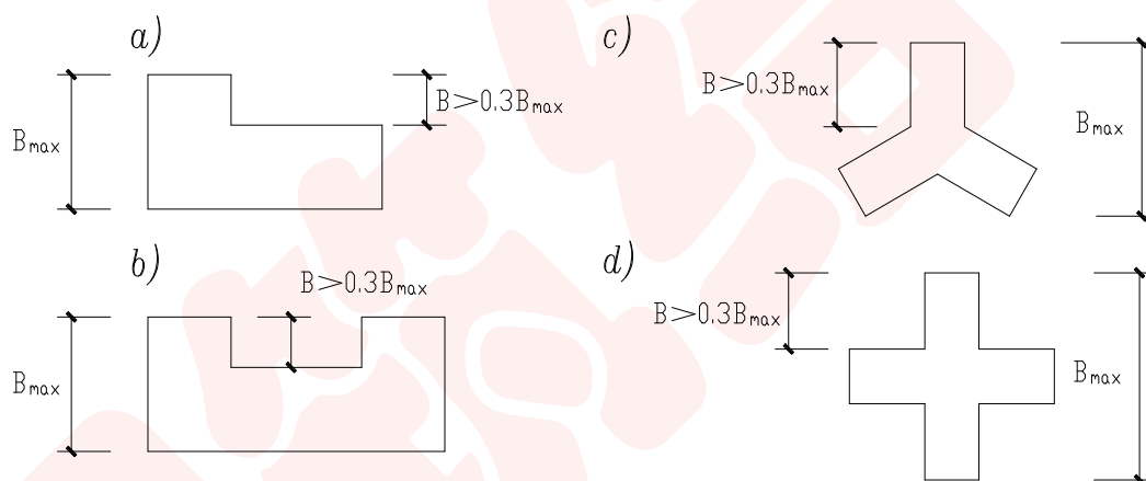
图 2 建筑结构平面的凸角或凹角不规则示例
