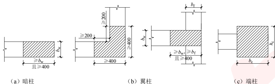
图 6.4.5-1 抗震墙的构造边缘构件范围
